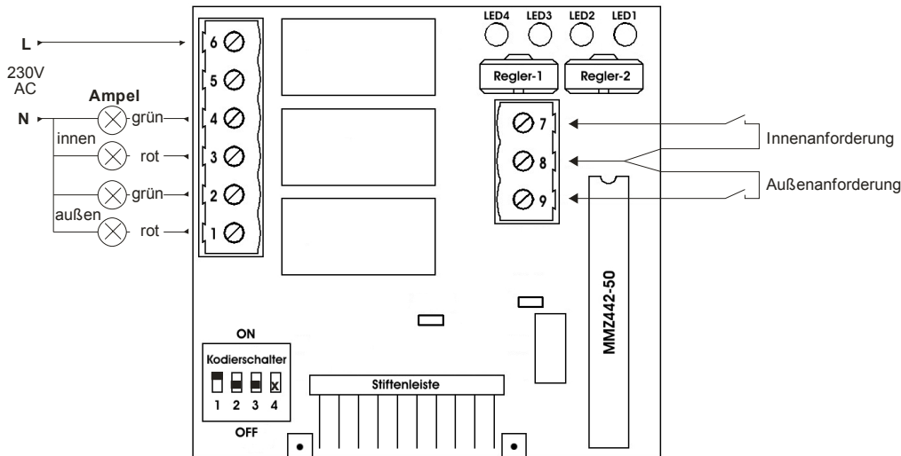
Schaltbild2:
