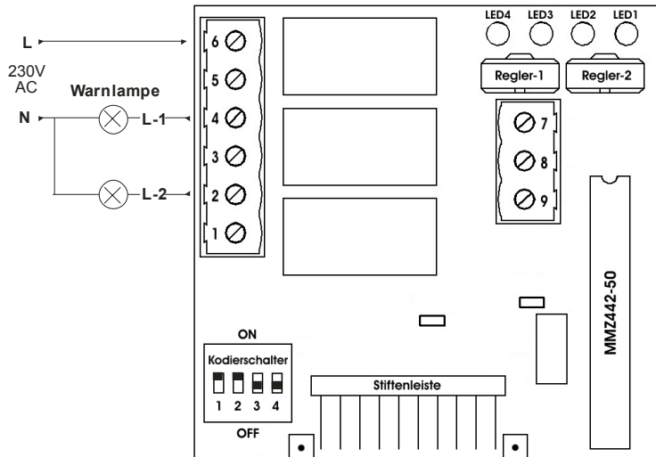
Schaltbild4:
