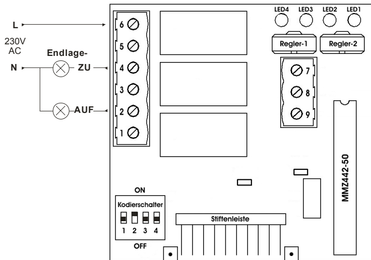
Schaltbild3:
